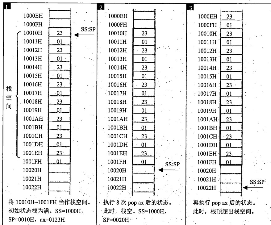
图 3.14 执行 pop 后栈顶超出栈空间
