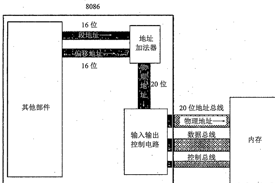
图 2.6 8086CPU 相关部件的逻辑结构
