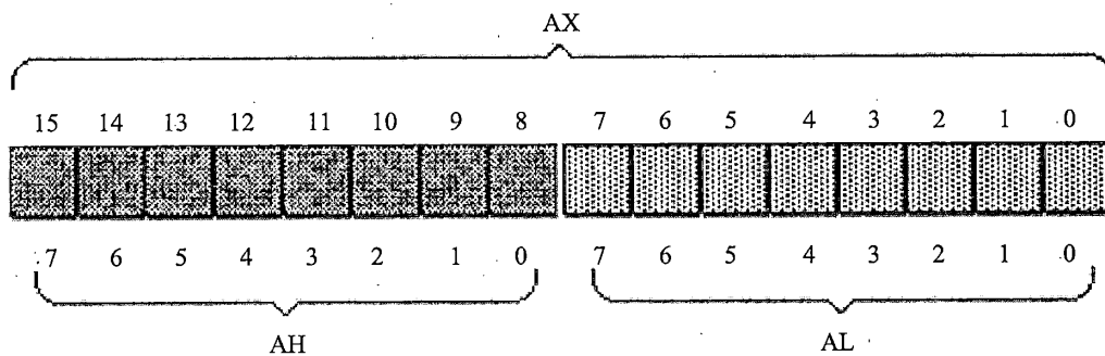
图 2.3 16 位寄存器分为两个 8 位寄存器
