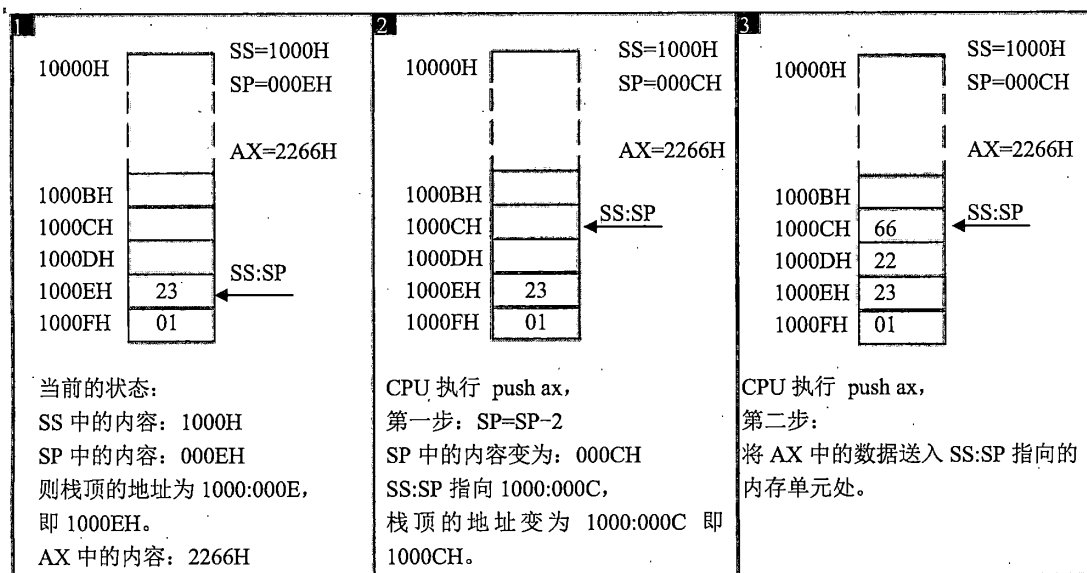
图 3.10 push 指令的执行过程
