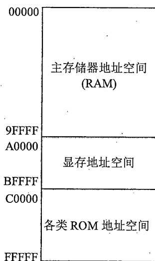
图 1.9 8086PC 机内存地址空间分配
