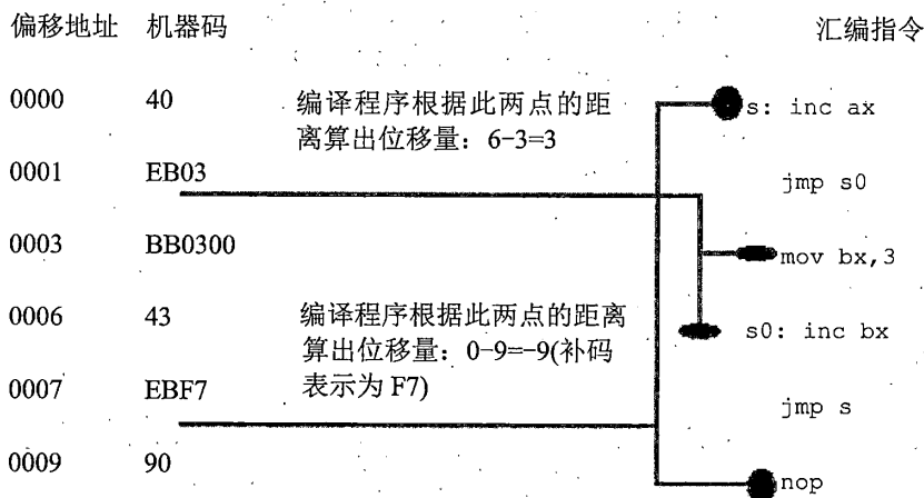
图 9.3 转移位移的计算方法
