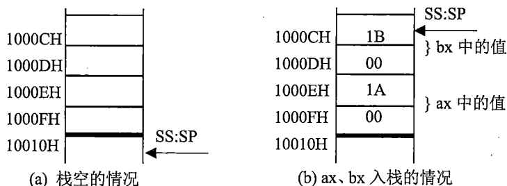
图 3.16 栈的情况示意(2)
