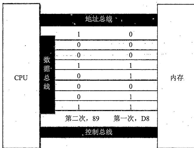
图 1.5 8 位数据总线上传送的信息
