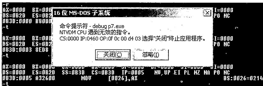
图 5.19 改写 0:0026 处存放的重要系统数据
