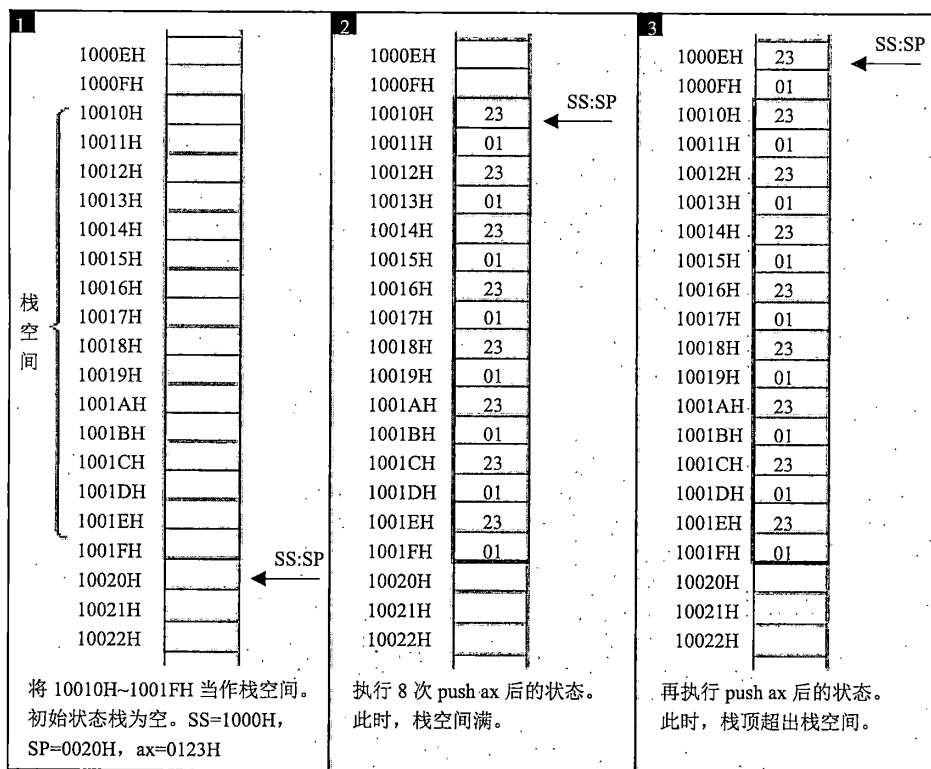
图 3.13 执行 push 后栈顶超出栈空间
