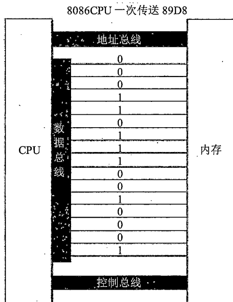
图 1.6 16 位数据总线上传送的信息
