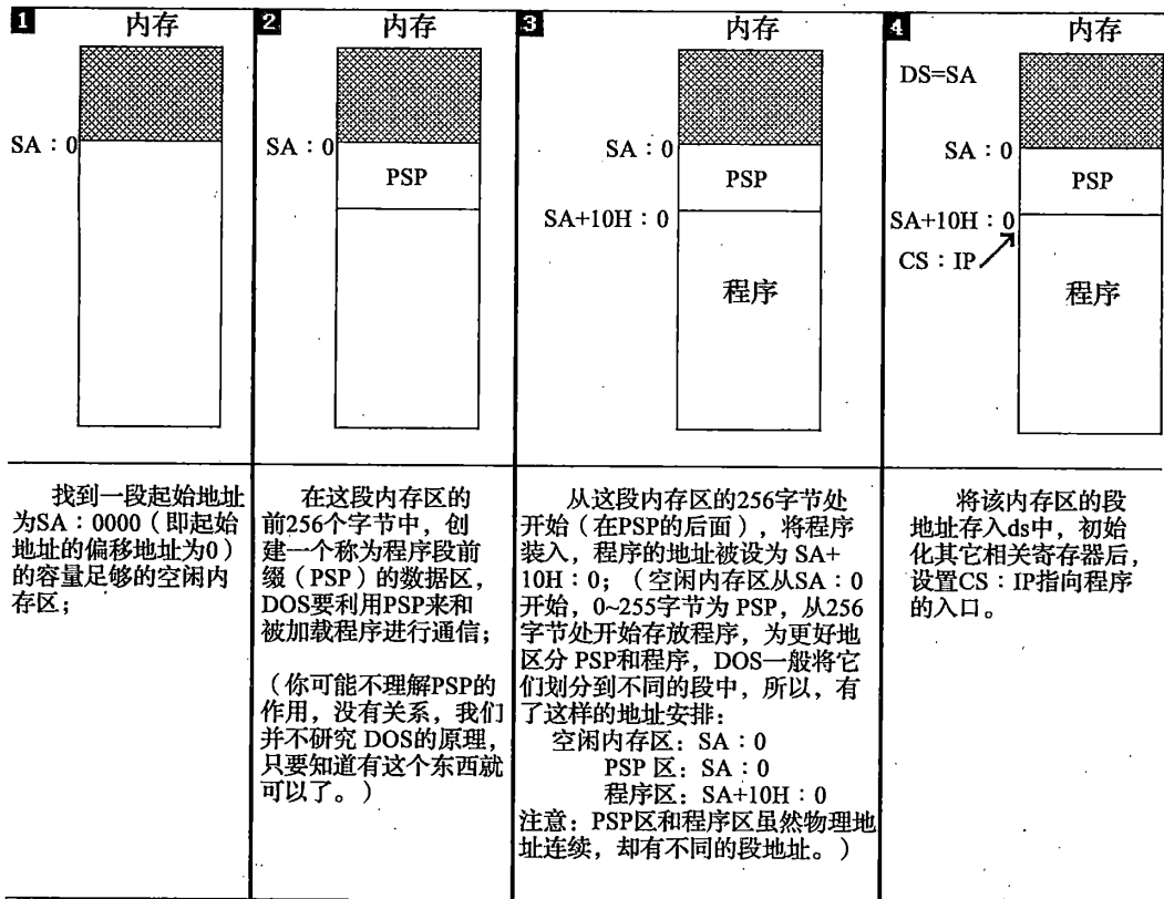
图 4.20 EXE 文件中程序的加载过程
