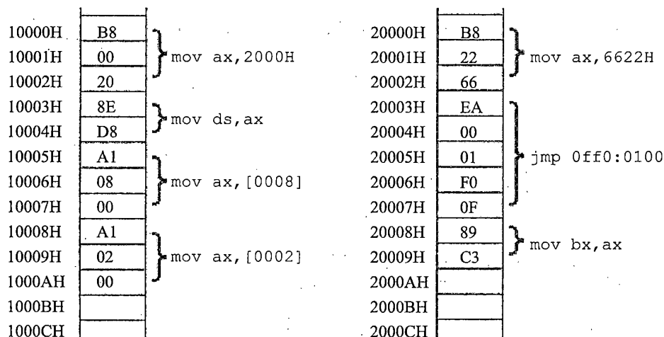
图 3.6 内存情况示意
