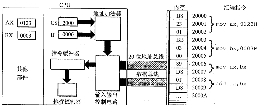
图 2.22 执行指令 BB 03 00(即 mov bx,0003H)
