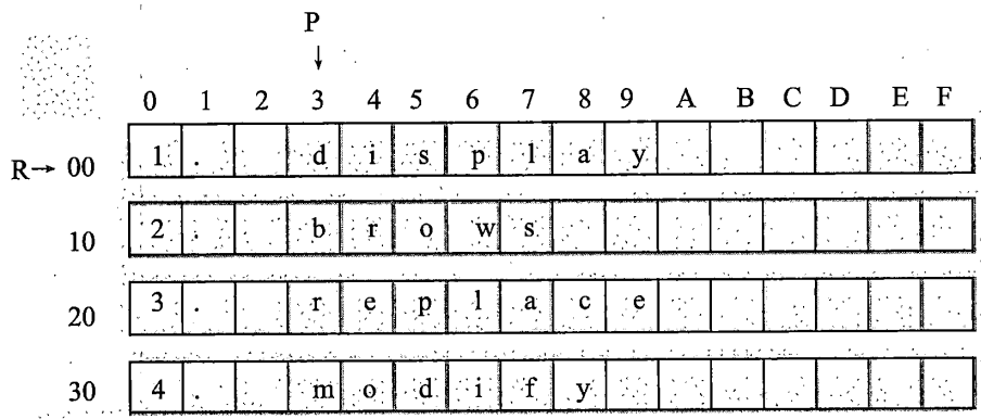
图 7.4 datasg 中数据的存储结构
