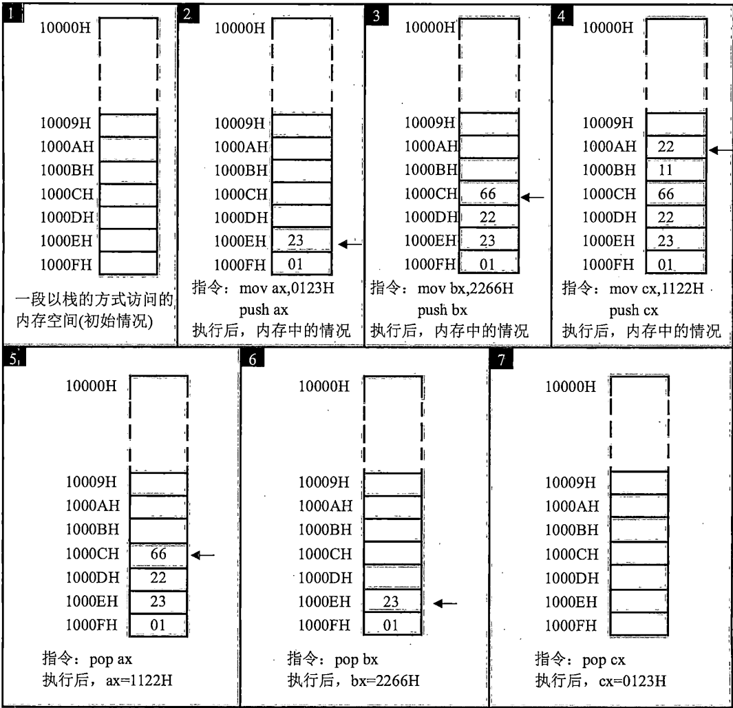
图 3.9 8086CPU 的栈操作
