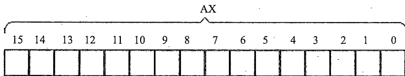
图 2.1 16 位寄存器的逻辑结构
