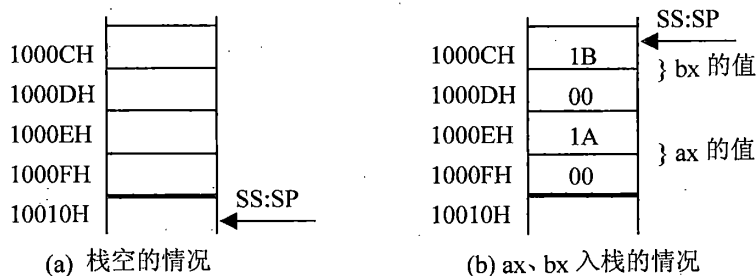
图 3.15 栈的情况示意(1)
