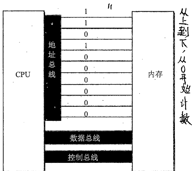
图 1.4 地址总线上发送的地址信息
