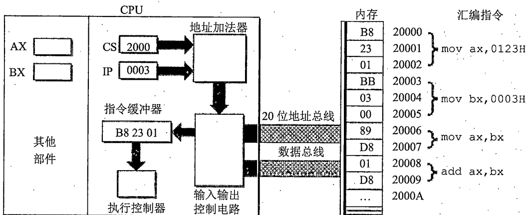
图 2.17 IP 中的值自动增加
