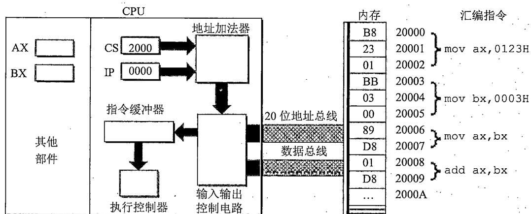
图 2.10 8086PC 读取和执行指令的相关部件
