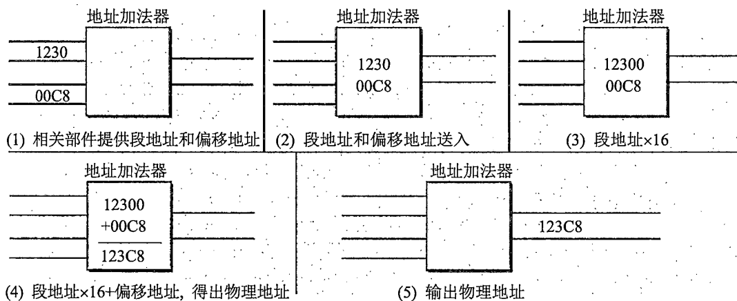
图 2.7 地址加法器的工作过程
