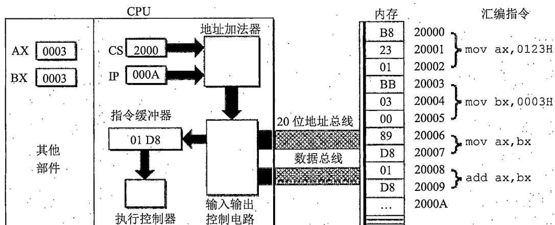
图 2.25 CPU 从内存 2008H 处读取指令 01 D8 入指令缓冲器(IP 中的值加 2)
