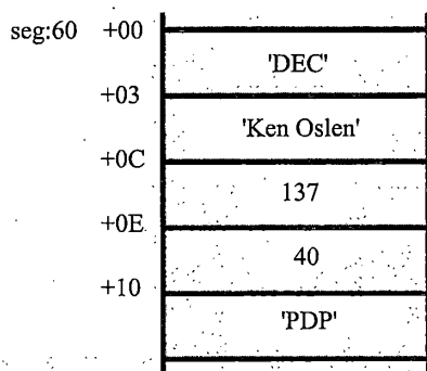
图 8.1 数据存放示意
