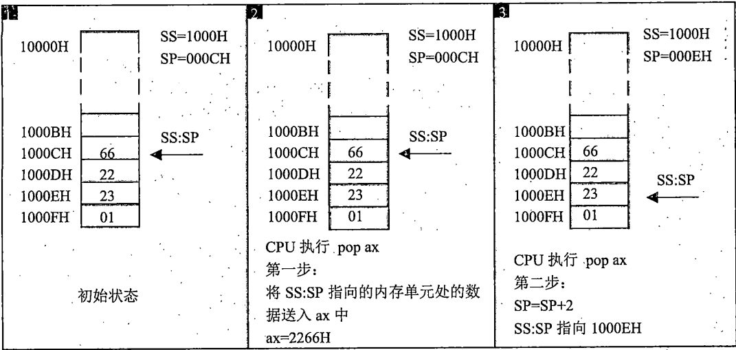
图 3.12 pop 指令的执行过程
