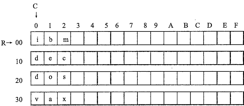
图 7.3 datasg 中数据的存储结构
