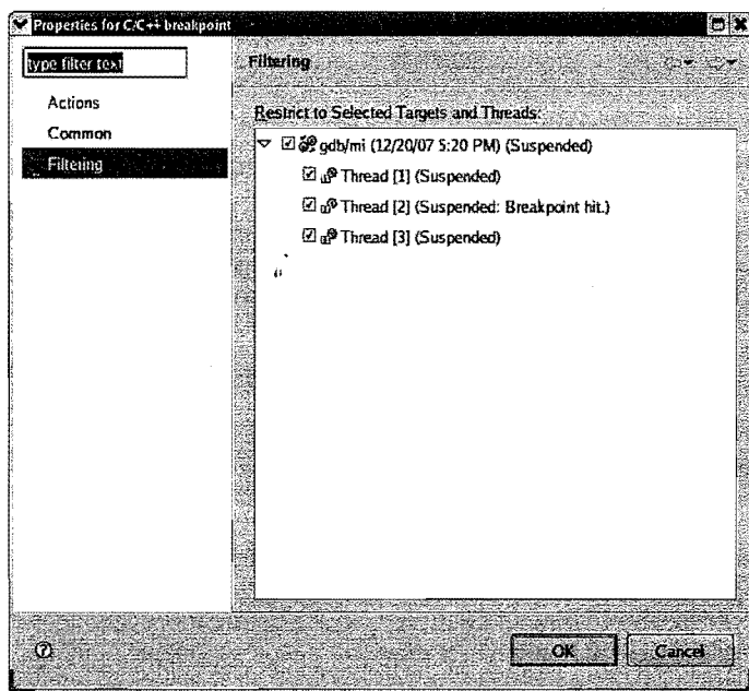
图5-3 在Eclipse中设置某个线程特有的断点
