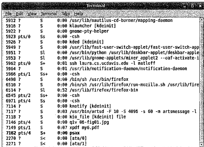
图6-1 某个终端窗口中的程序运行情况
