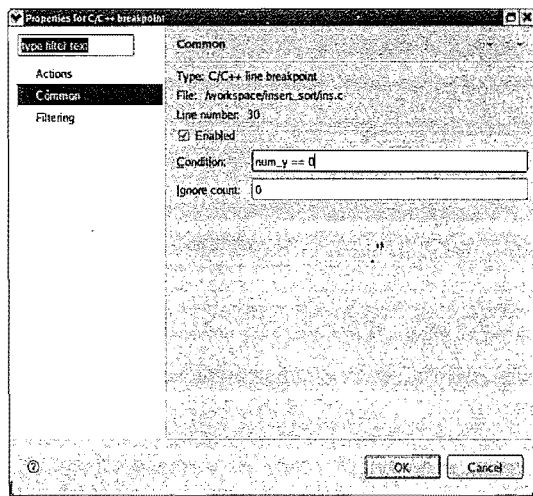
图1-16 使断点成为条件断点
