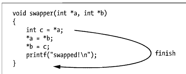
图2-11 finish恢复执行，直到当前函数返回为止
