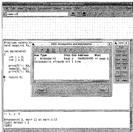
图2-4 两个被删除的断点
