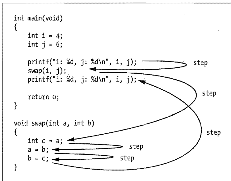
图2-8 step单步进入函数
