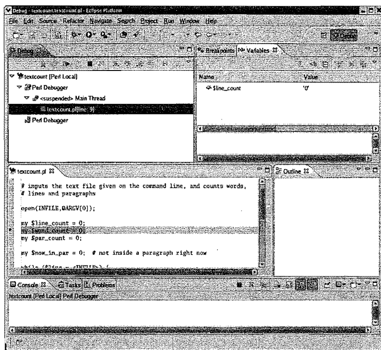
图8-5 Perl调试屏幕
