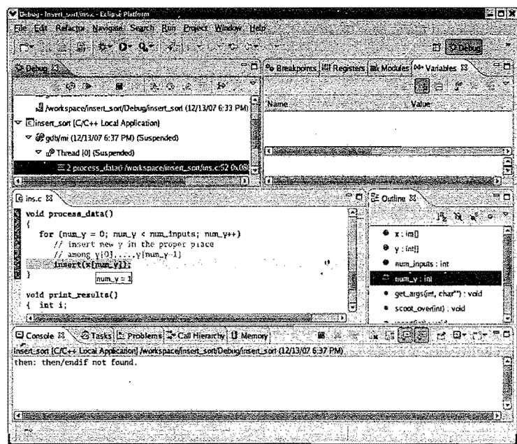
图1-6 在Eclipse中查看变量
