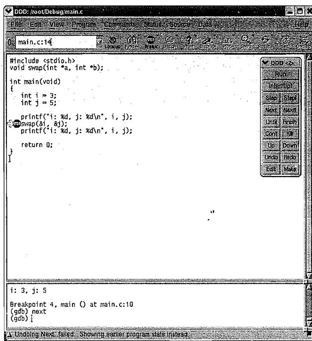
图2-14 单击Undo撤销上一个操作
