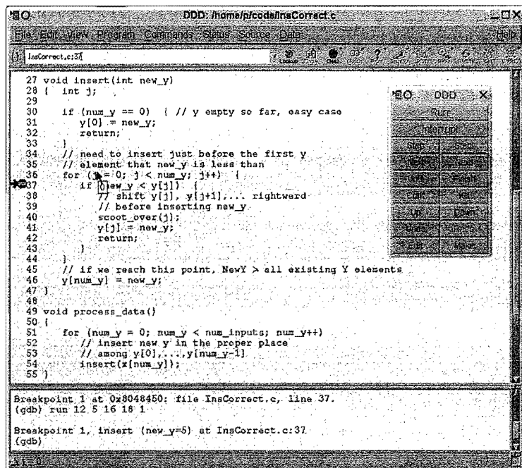
图1-5 在DDD中查看变量
