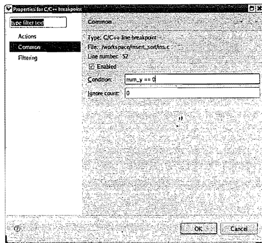
图2-17 在Eclipse中对断点施加条件
