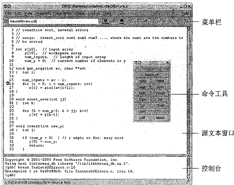
图1-1 DDD布局
