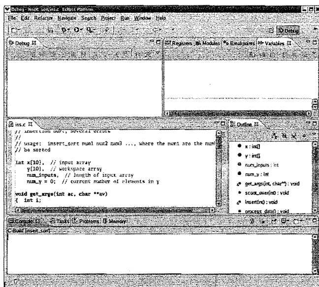
图1-3 Eclipse环境
