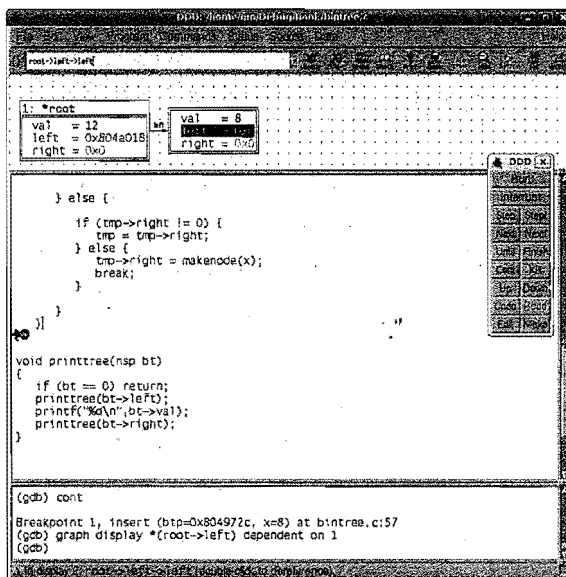
图3-3 跟踪链接
