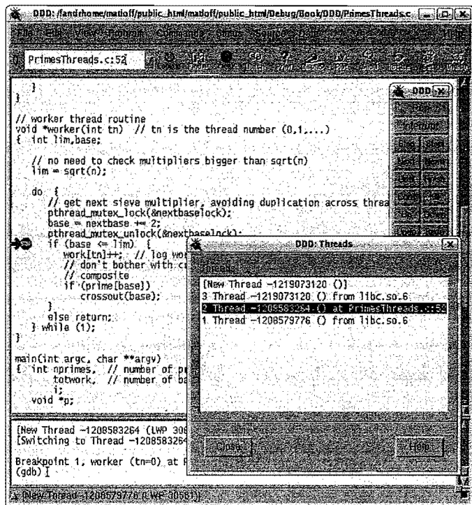
图5-1 线程窗口
