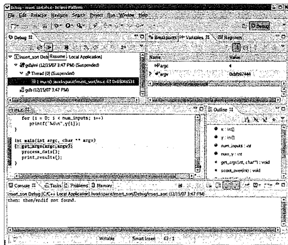
图1-13 调试运行的开始
