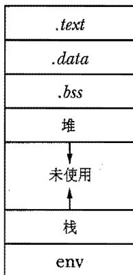
图4-1 程序内存布局
