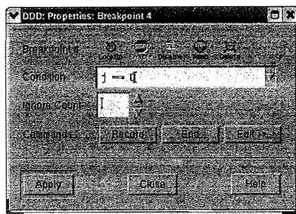
图2-16 在DDD中对断点施加条件
