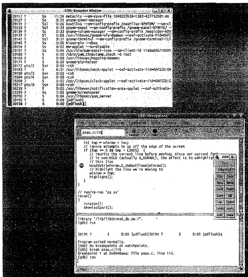
图6-2 在DDD中附加到运行程序上
