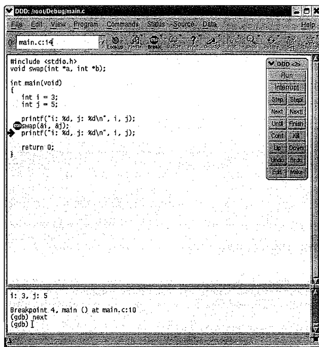
图2-13 不小心按了Next按钮
