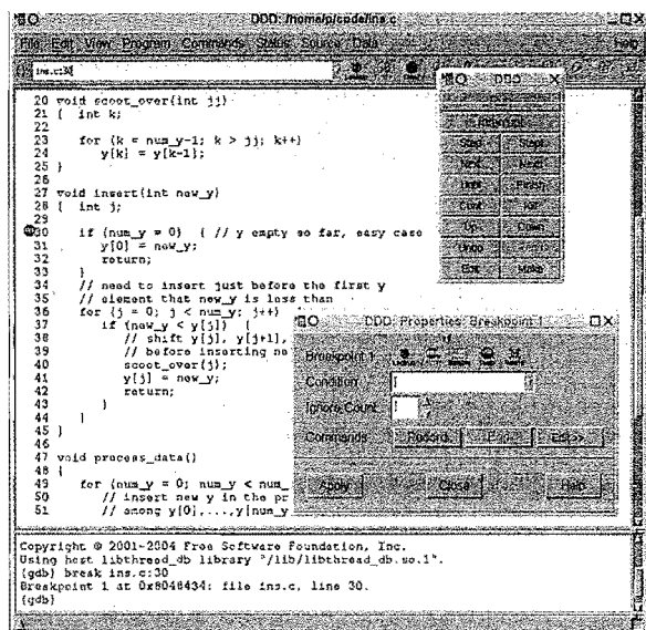
图1-11 在断点上施加一个条件
