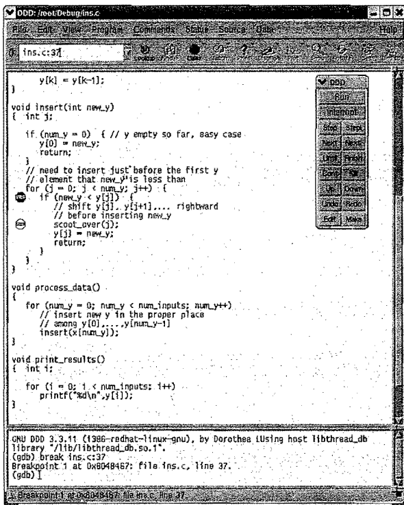
图2-6 在DDD中“移动”断点
