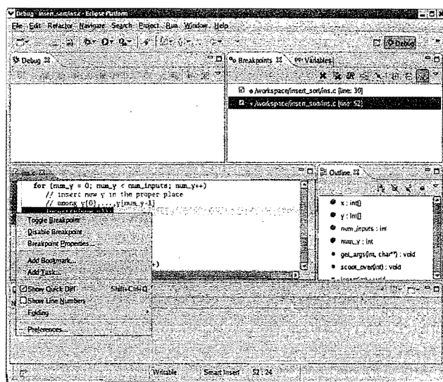
图2-5 在Eclipse中删除/禁用断点
