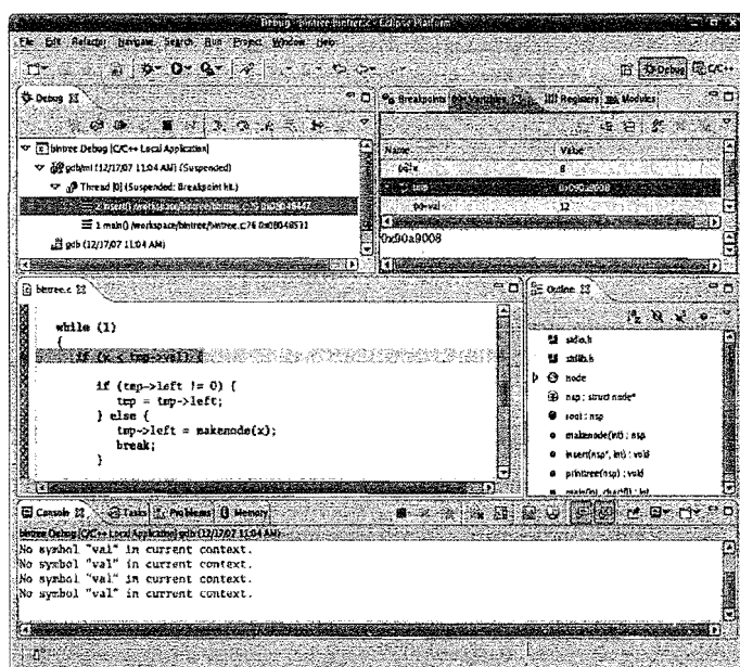
图3-5 在Eclipse中检查struct字段
