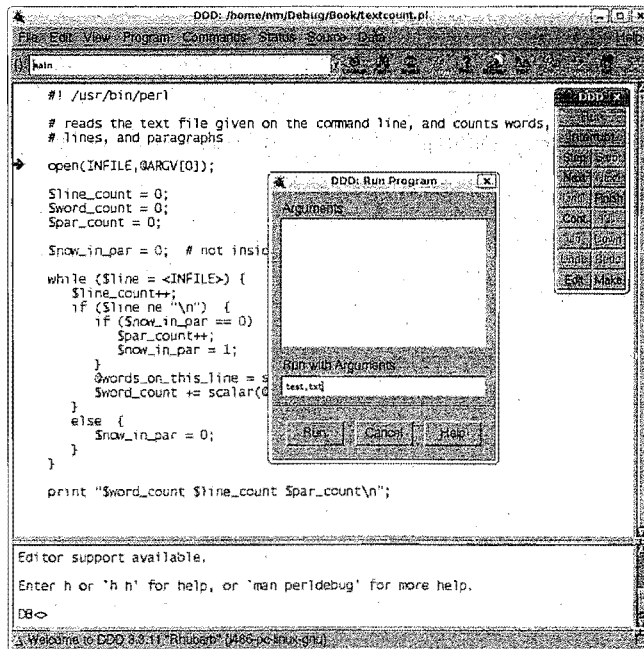
图8-2 设置命令行参数
