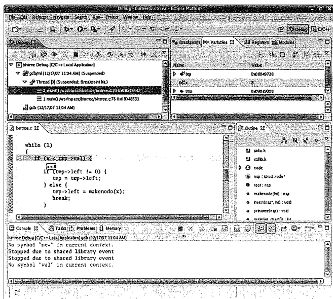
图3-4 在Eclipse中检查标量变量
