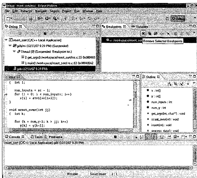
图1-4 在Eclipse中删除断点
