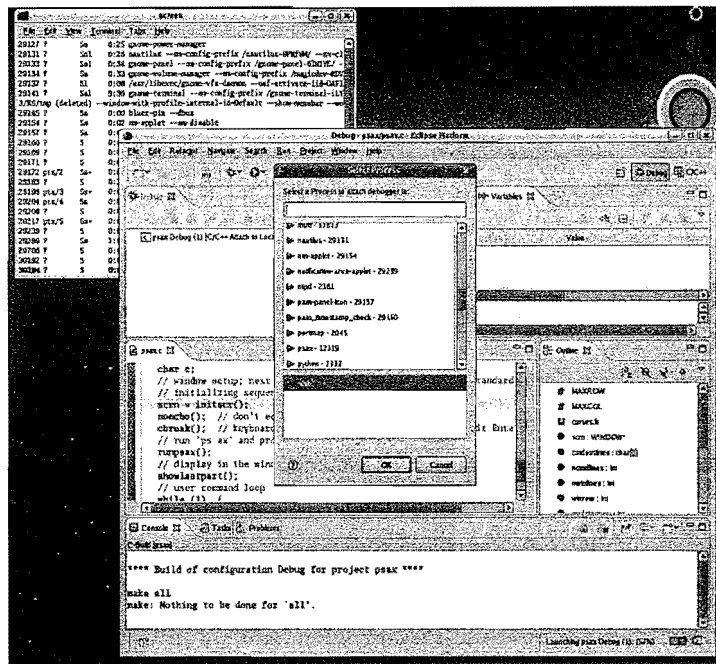
图6-4 选择要将GDB附加到的进程
