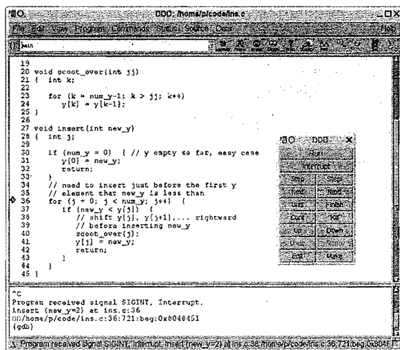
图1-9 中断后的屏幕
