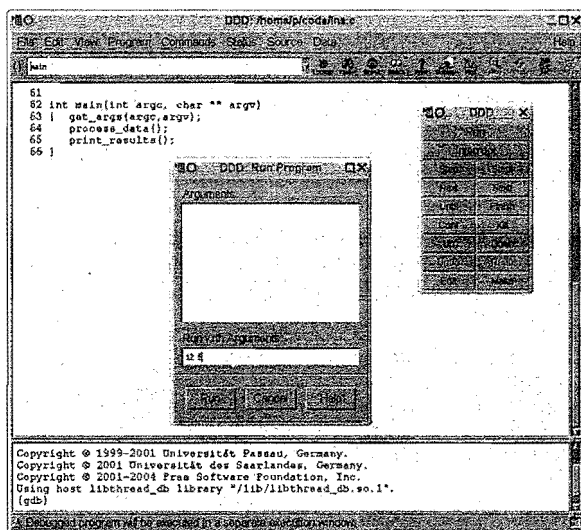
图1-8 DDD的Run命令
