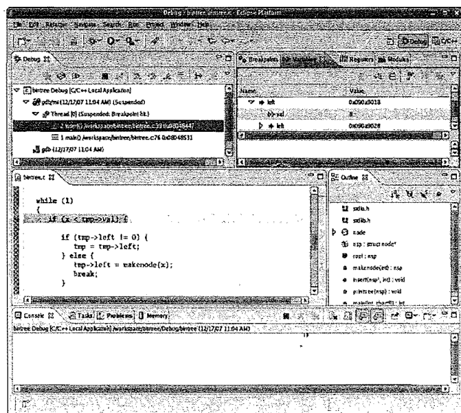
图3-6 在Eclipse中跟踪指针链接
