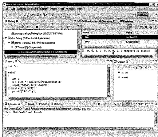
图3-7 在Eclipse中显示一个动态数组
