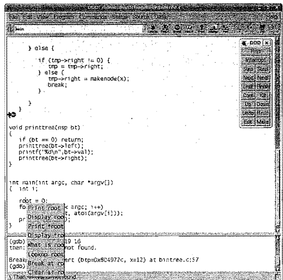
图3-1 查看变量的弹出窗口
