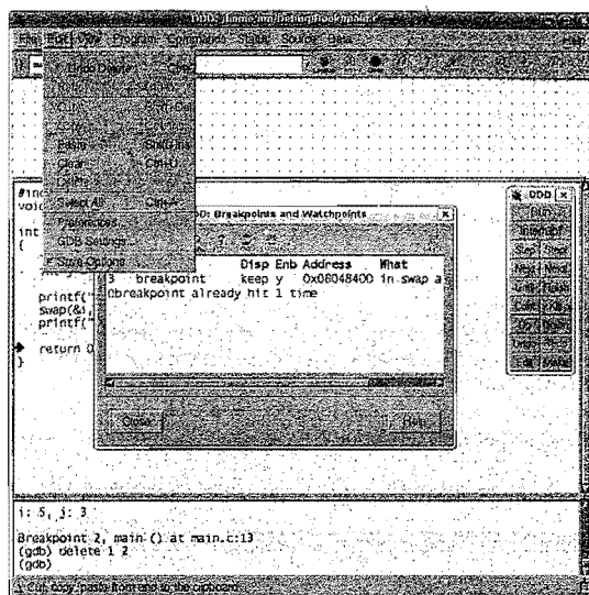
图2-7 DDD中恢复两个断点的机会
