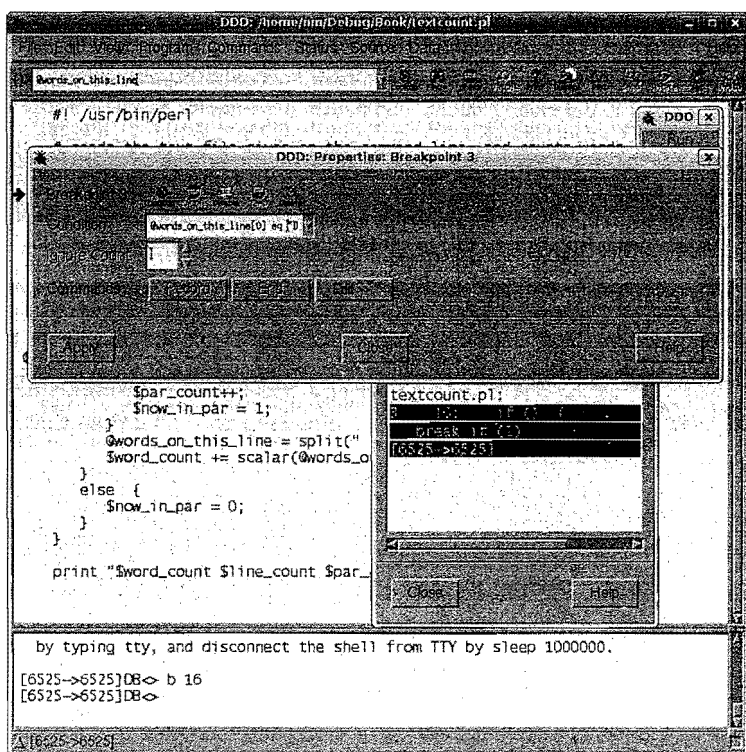
图8-3 在断点上设置条件
