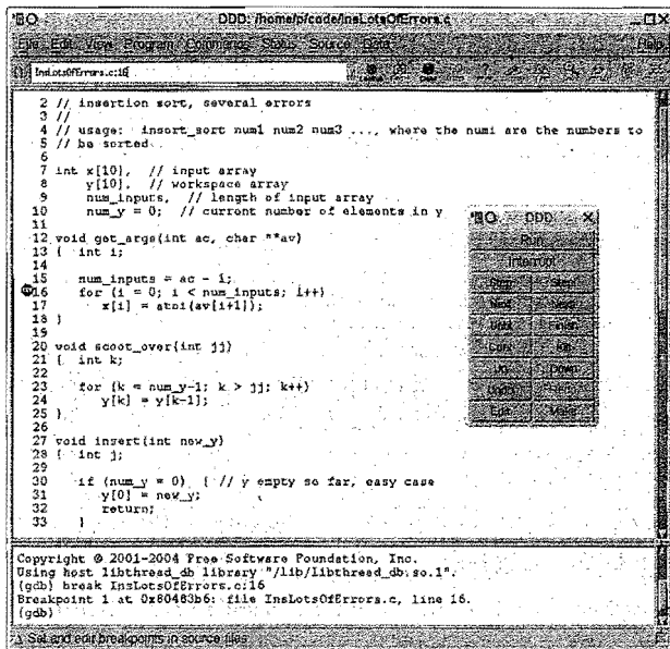
图1-2 断点设置
