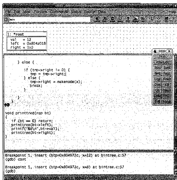
图3-2 节点的显示
