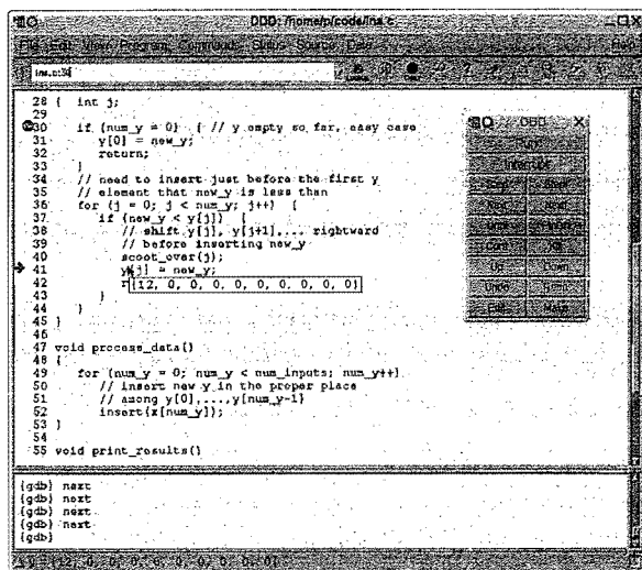
图1-10 检查数组
