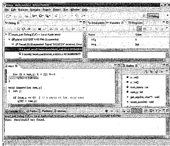
图1-15 段错误
