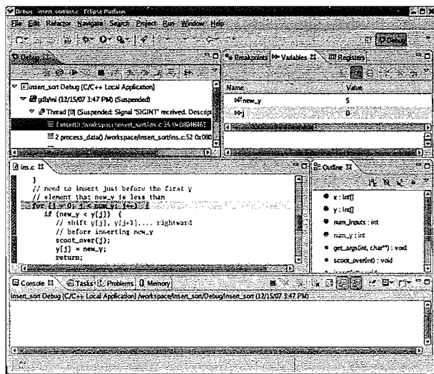
图1-14 挂起的程序
