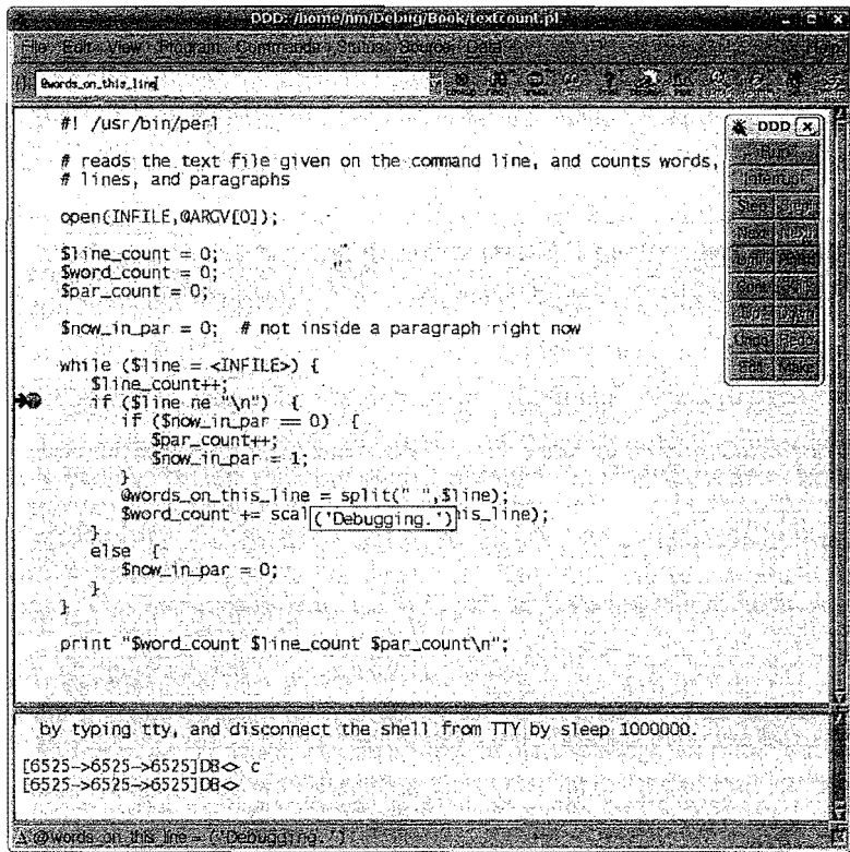
图8-4 到达断点时的情况
