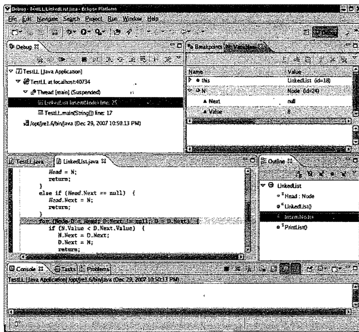
图8-1 Eclipse中的Java调试
