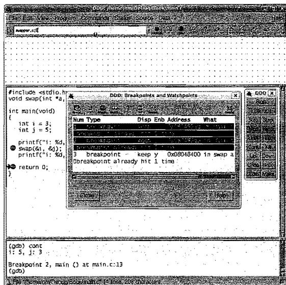
图2-3 在DDD中删除/禁用/启用多个断点
