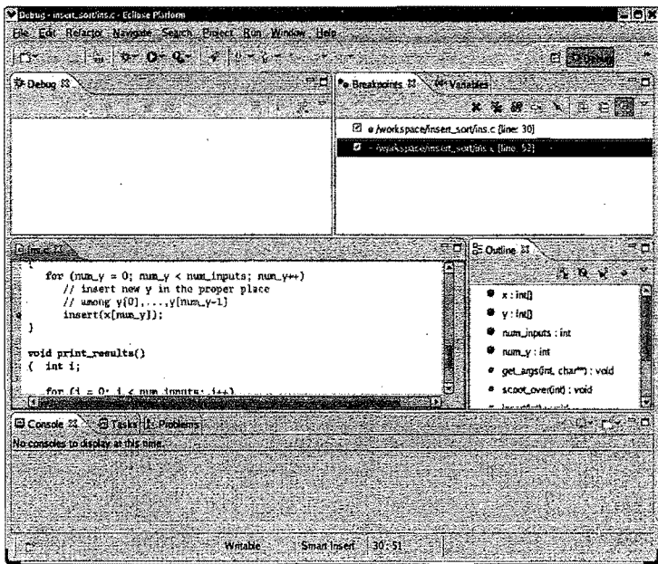
图2-2 在Eclipse中查看断点
