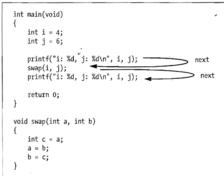
图2-9 next单步越过函数
