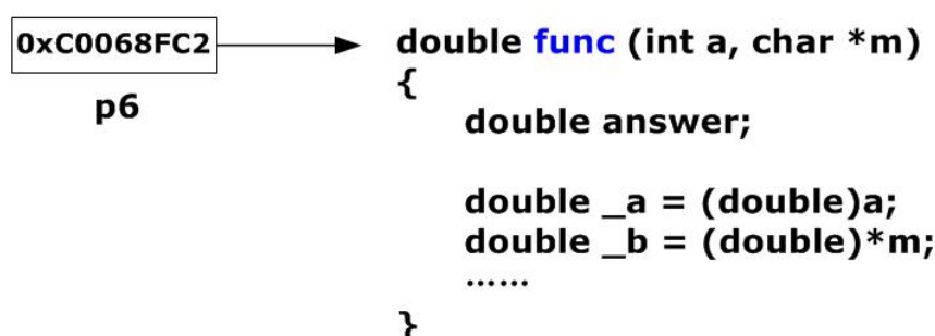
图 2-47 指向函数的指针
