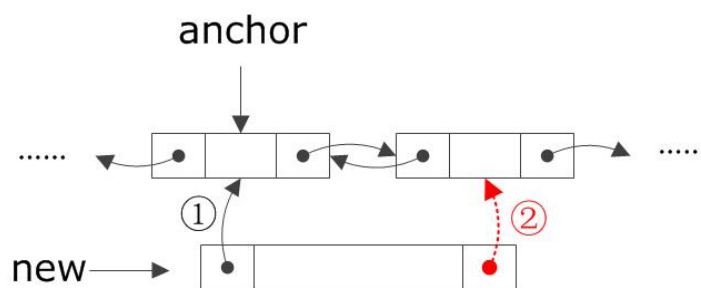
图 3-16 双向循环链表节点的前插操作（2）
