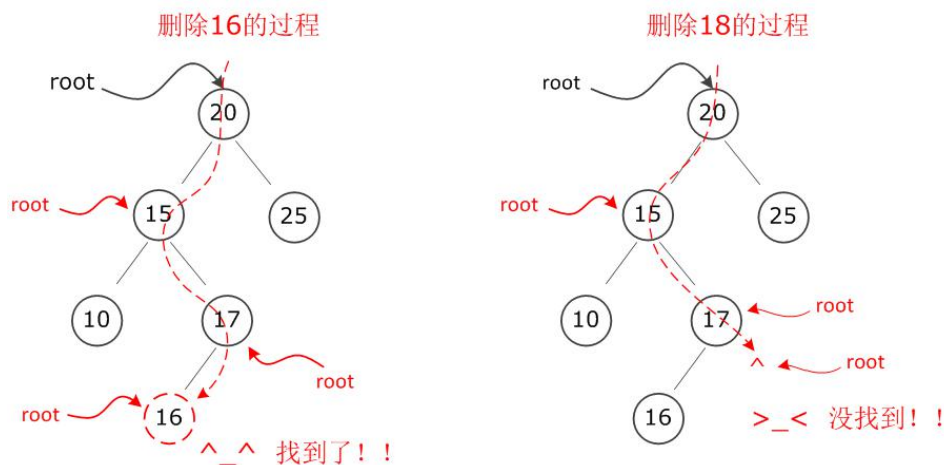
图3-63 根节点的相对性
