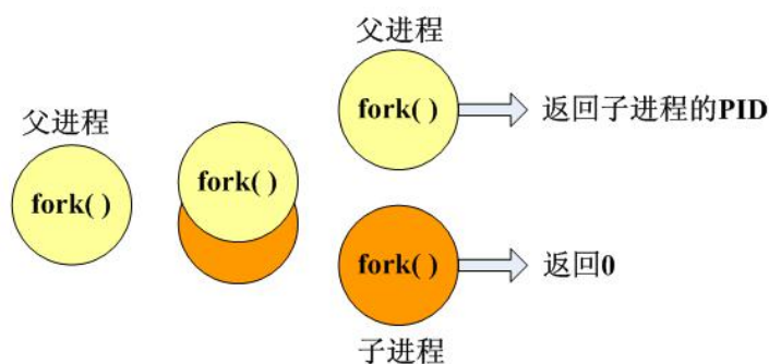
图 5-4 创建子进程的过程示意图
