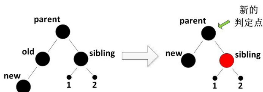
图 3-94 黑父 + 双黑侄的操作
