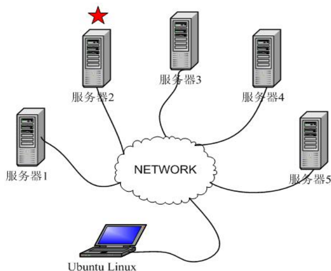
图1-14 APT 软件管理拓扑结构
