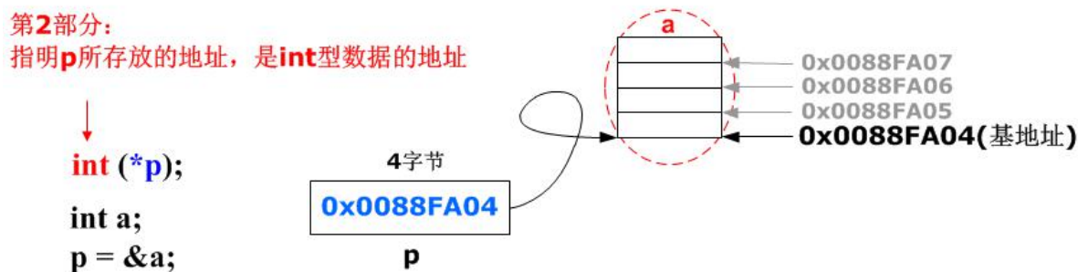
图 2-42 指针定义——第 2 部分
