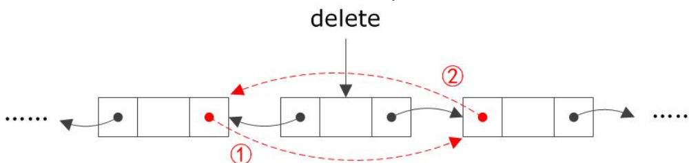
图 3-23 双向循环链表节点的删除操作（1）
