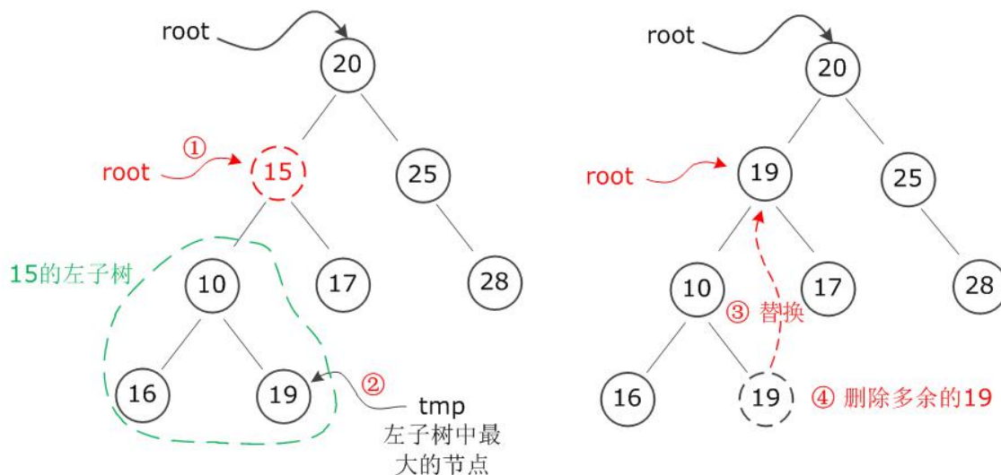
图3-62 BST 的删除算法（一）
