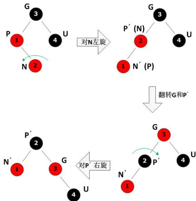
图 3-84 插入节点 N 时 P 为红色且 U 为黑色（情形一）
