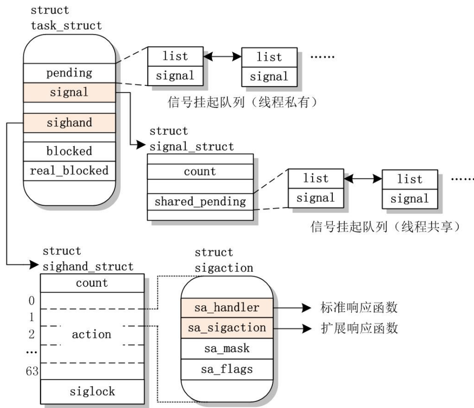
图 5-7 内核中跟信号处理相关的数据结构
