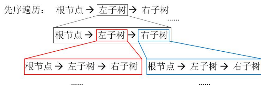
图 3-68 先序遍历的逻辑
