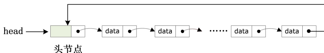
图 3-10 单向循环链表
