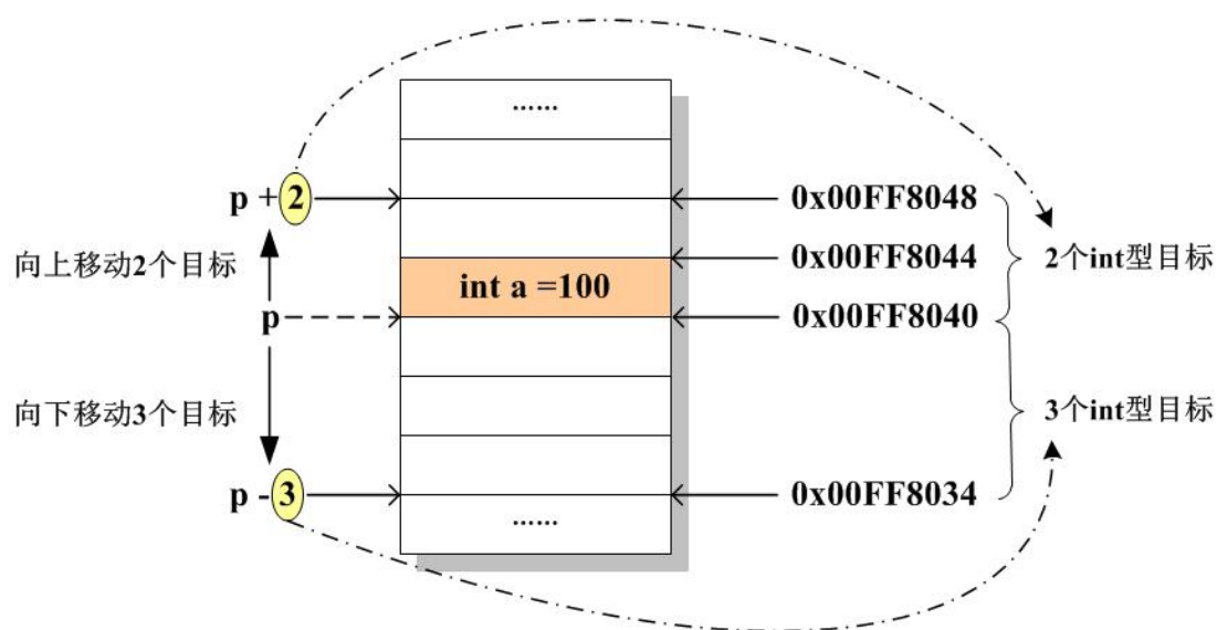
图 2-49 指针的加减法
