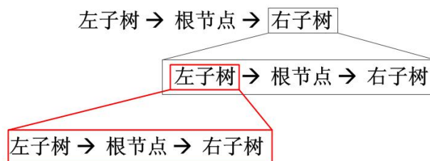
图 3-69 中序遍历的逻辑
