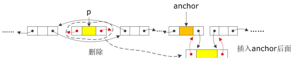
图 3-25 双向循环链表节点的移动操作（1）
