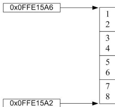
图 2-14 一个整型变量 0x12345678
