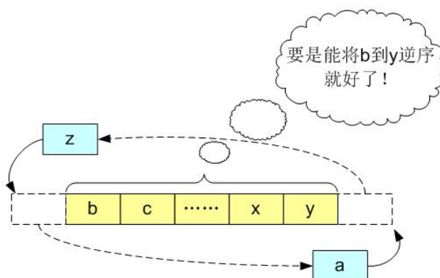
图 2-23 逆转一个字符串
