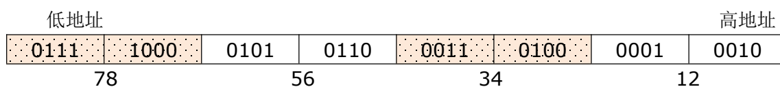
图 2-3 正整数的二进制真实内存存储视图（以小端序为例）
