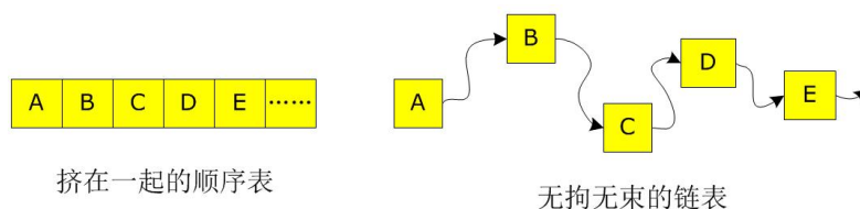
图 3-2 顺序表和链表
