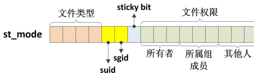
图 4-9 st_mode 内部结构
