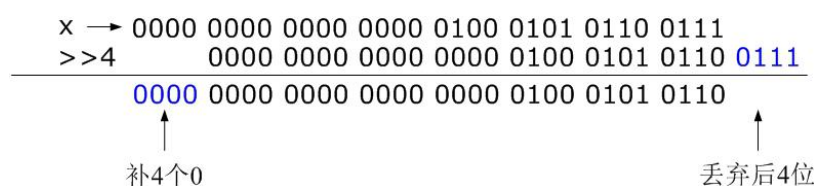
图 2-11 右移运算
