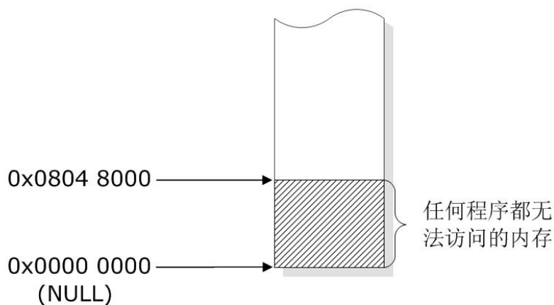
图 2-44 空指针
