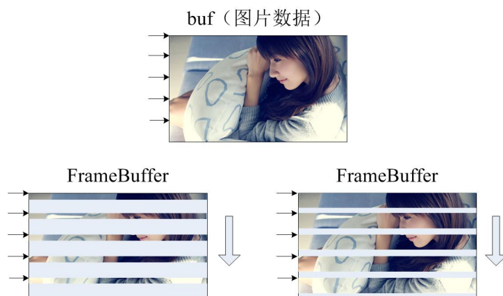
图 6-21 百叶窗效果
