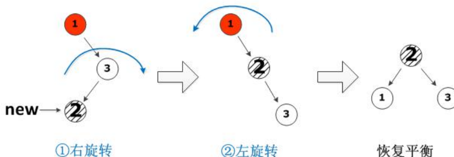
图 3-79 右-左旋转
