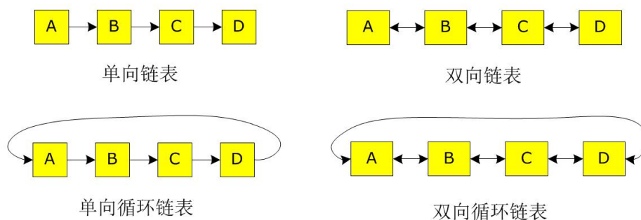
图 3-3 各种链表
