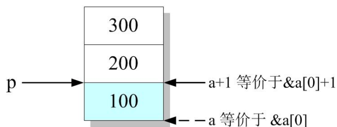
图 2-50 数组的运算
