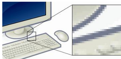
图 6-10 像素点
