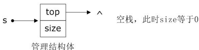
图 3-44 空的链式栈
