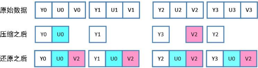
图 6-27 YUV411
