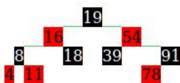
图 3-82 红黑树
