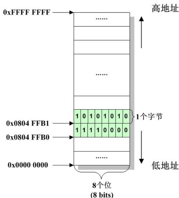
图 2-37 内存景色
