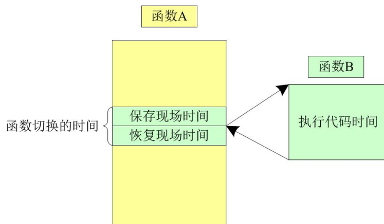
图 2-30 函数的切换
