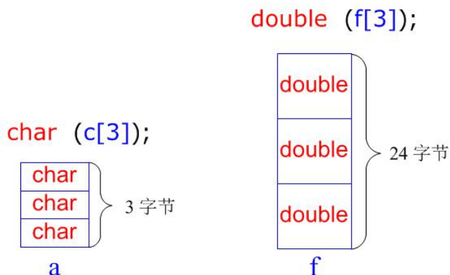
图 2-35 各种数组
