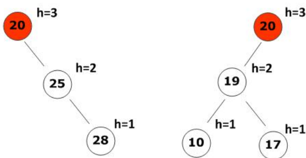
图 3-73 非平衡树
