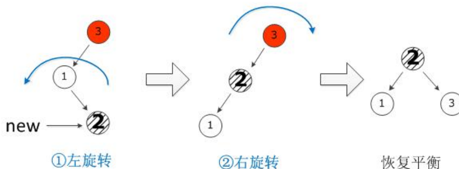
图 3-78 左-右旋转
