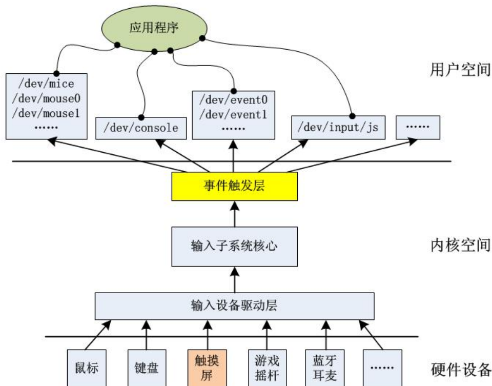
图 4-12 输入子系统
