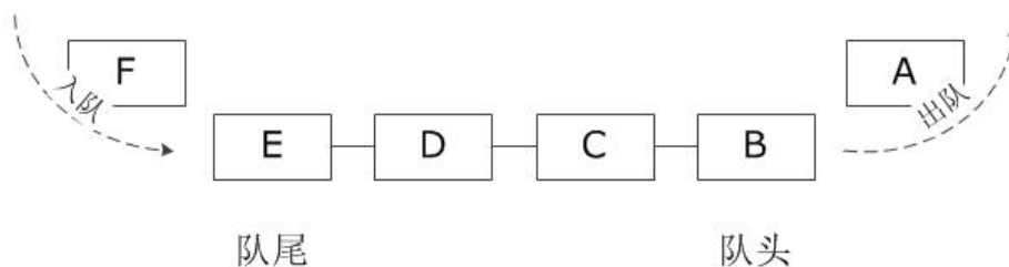
图 3-49 队列的逻辑
