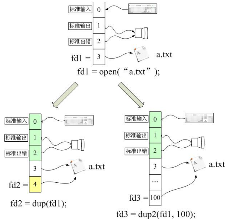
图 4-7 dup( )与 dup2( )
