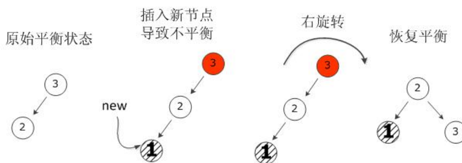
图 3-75 右旋转
