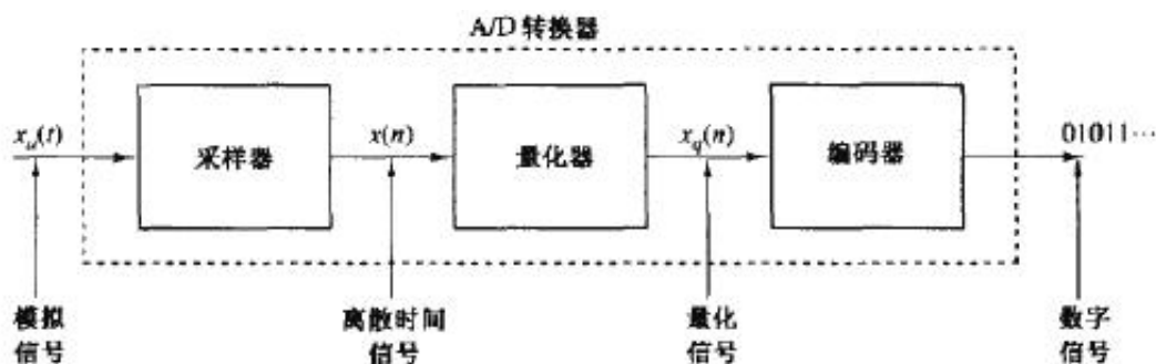
图 6-1 数模转换
