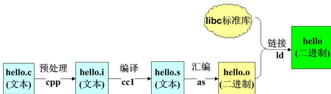
图 1-35 编译过程
