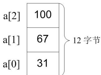
图 2-36 数组的下标
