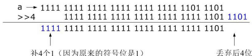
图 2-13 算术右移
