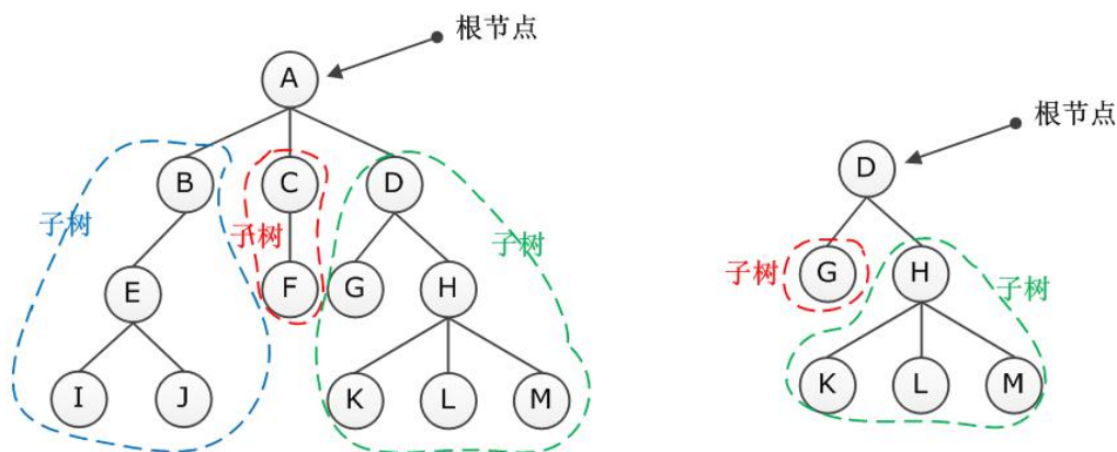
图 3-56 树和子树
