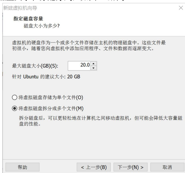
图1-6 选择磁盘
