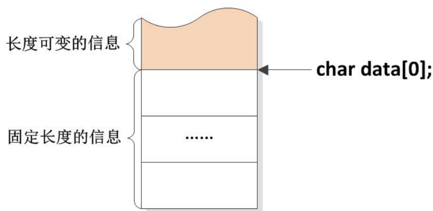
图 2-53 柔性数组
