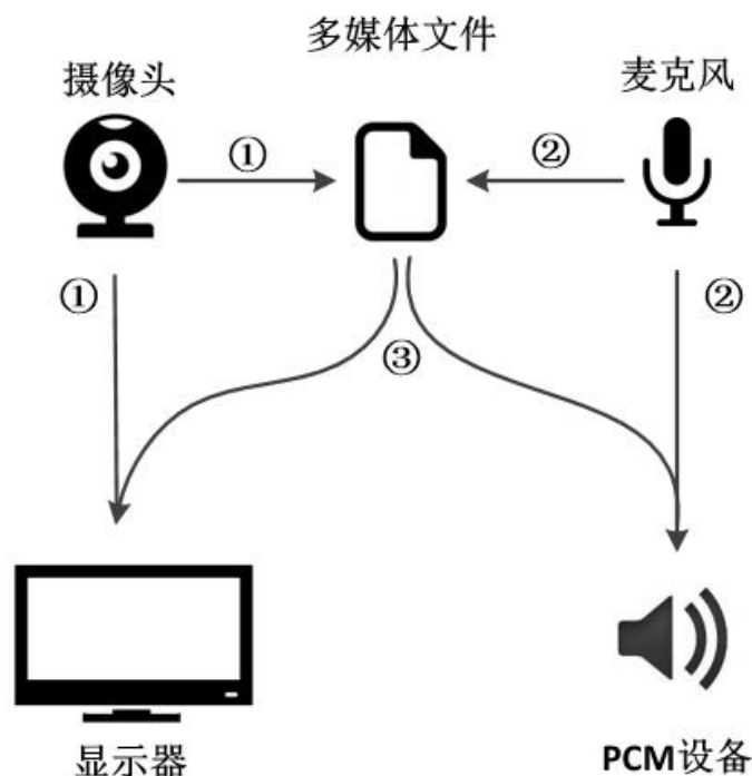
图 6-24 媒体流
