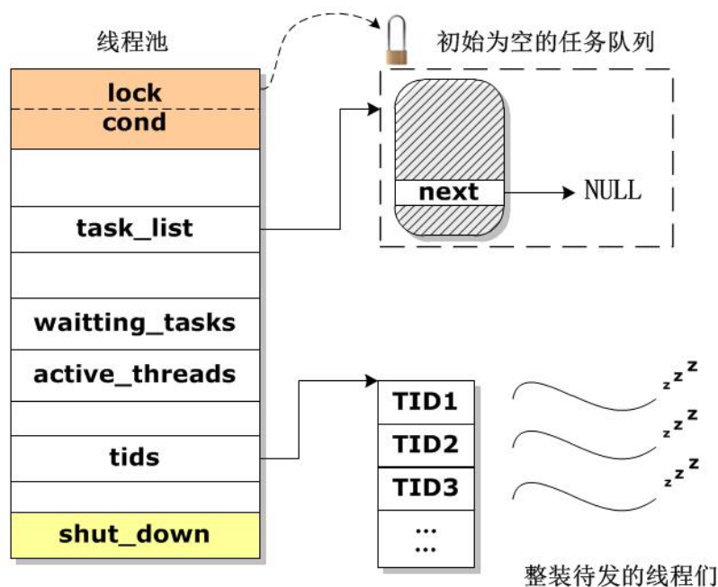
图 5-20 线程池
