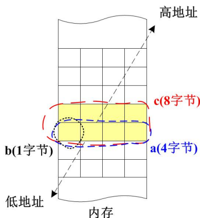
图 2-65 联合体
