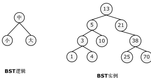
图 3-59 BST 示例
