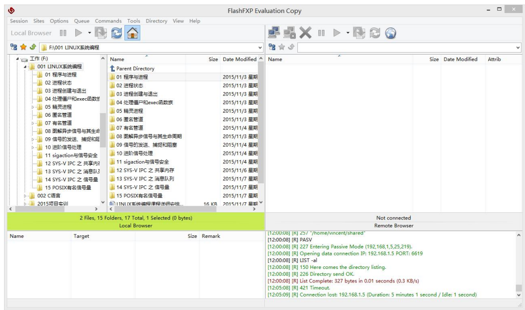
图 1-22 FlashFXP
