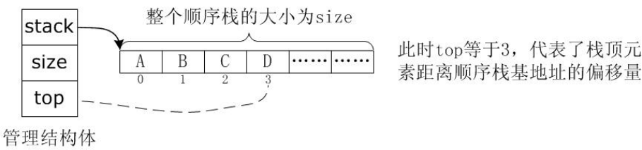
图 3-43 顺序栈
