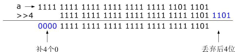
图 2-12 逻辑右移
