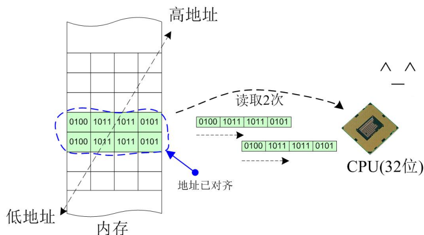
图 2-63 地址对齐的数据
