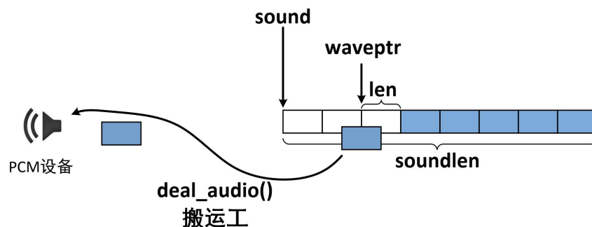
图 6-35 音频数据处理流程
