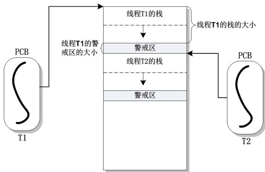
图 5-17 进程中各个线程相对独立的栈
