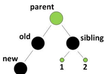
图 3-92 old 的兄弟为黑色
