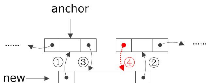
图 3-18 双向循环链表节点的前插操作（4）
