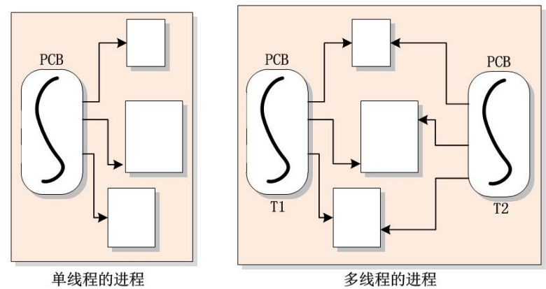
图 5-16 进程中的线程
