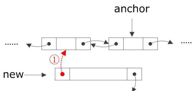
图 3-19 双向循环链表节点的后插操作（1）
