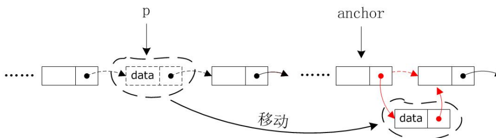
图 3-9 单向链表中节点的移动
