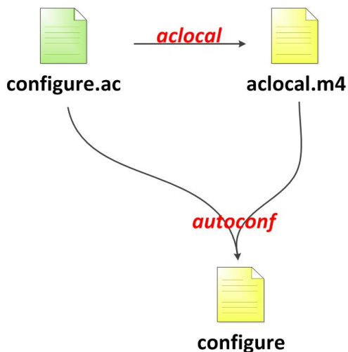
图 1-41 从 configure.ac 生成的文件
