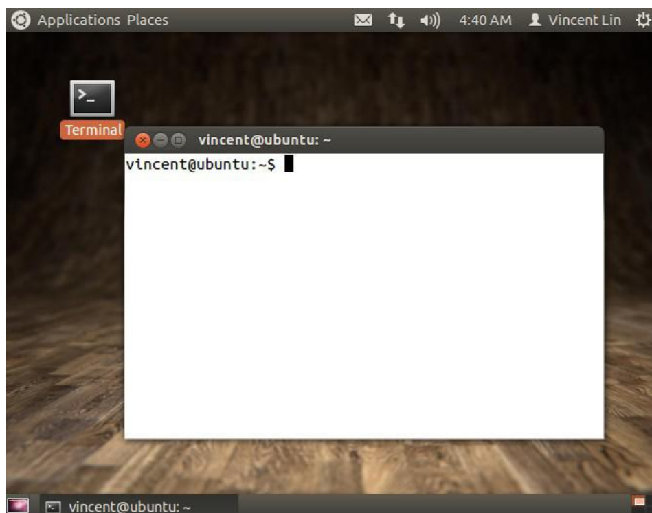
图 1-24 Linux 伪终端
