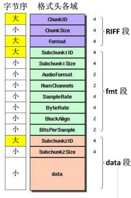
图 6-6 WAVE 格式头
