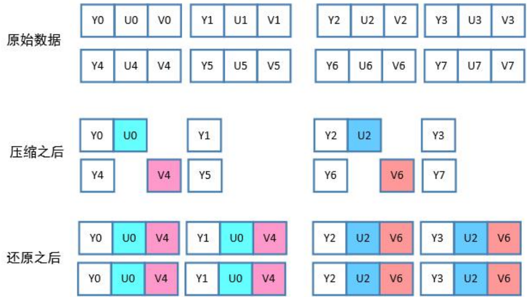
图 6-28 YUV420
