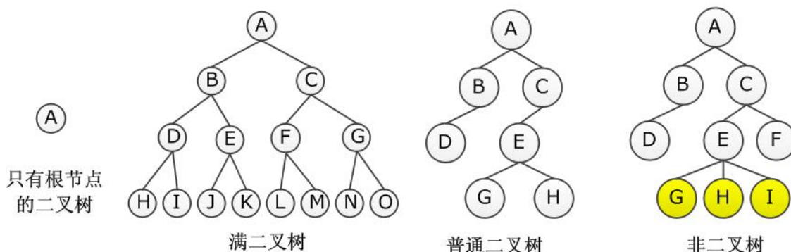
图 3-57 各种二叉树
