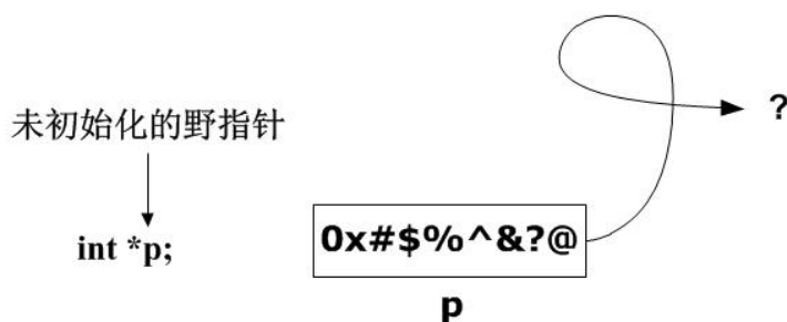
图 2-43 野指针
