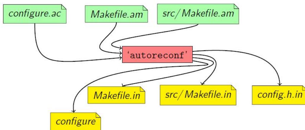
图1-43 autoreconf的作用
