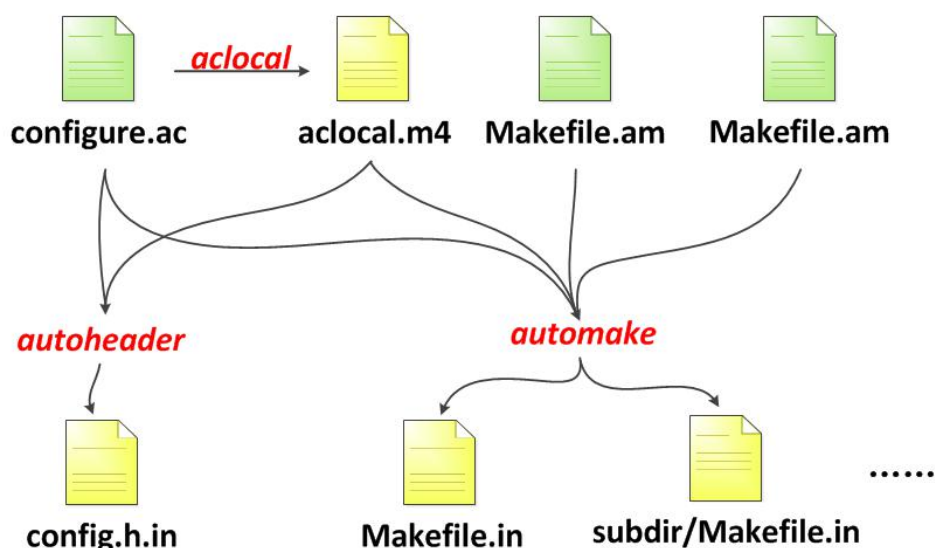
图 1-42 autoheader 和 automake
