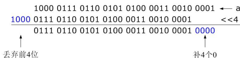
图 2-10 左移运算
