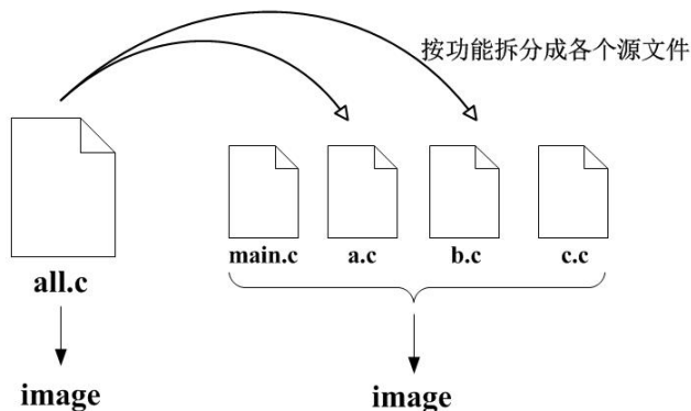
图 2-66 多文件编译
