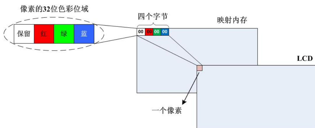
图 6-14 色彩深度
