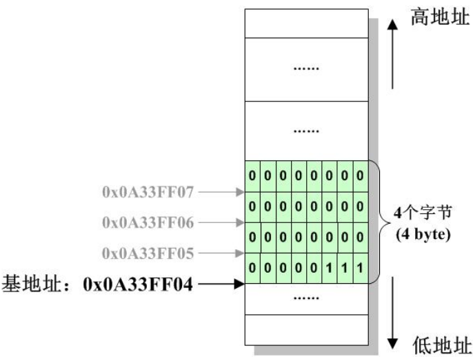
图 2-38 字节与地址
