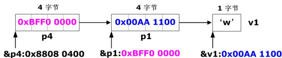
图 2-45 多级指针
