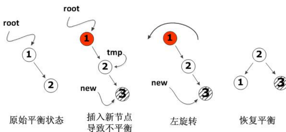
图 3-77 左旋转
