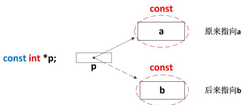
图 2-55 const 型指针
