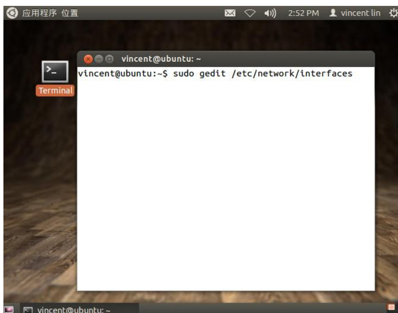
图 1-13 Linux 伪终端
