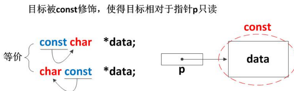
图 2-54 const 型指针
