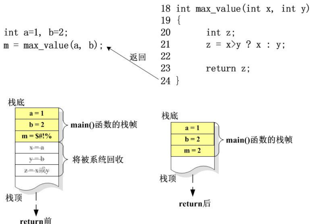
图 2-21 函数的返回
