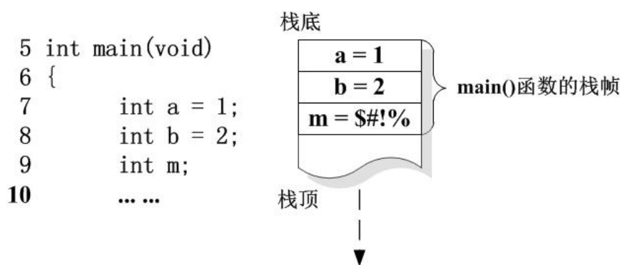
图 2-19 函数的栈帧
