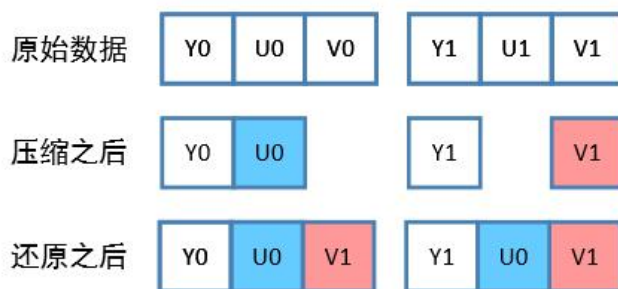
图 6-26 YUV422
