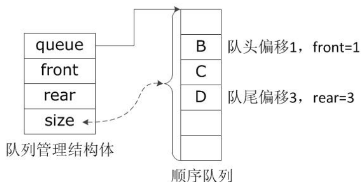
图 3-50 顺序队列
