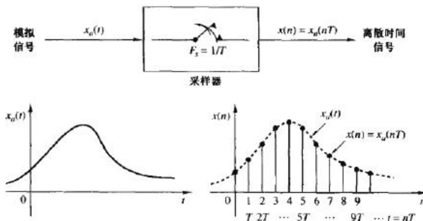
图 6-2 采样
