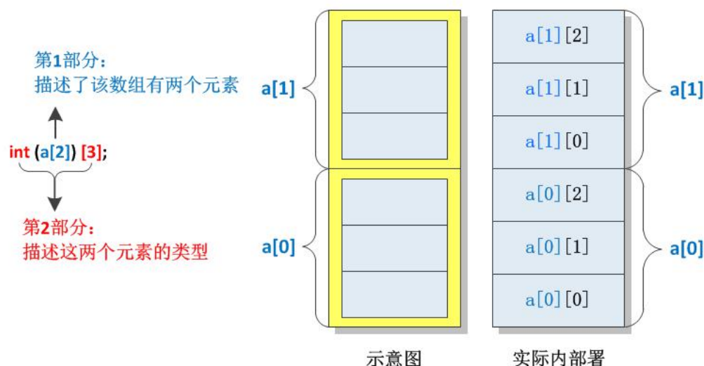
图 2-51 二维数组
