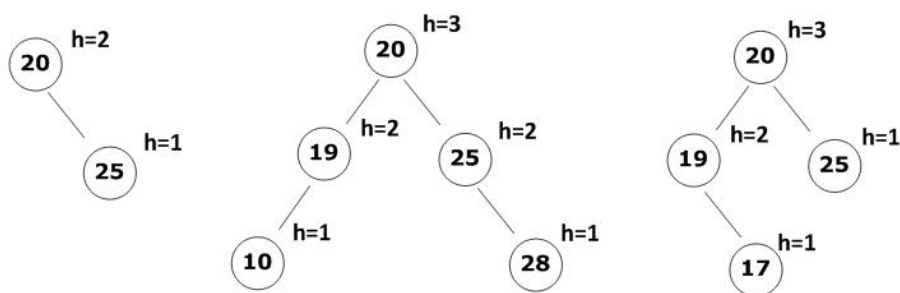
图 3-72 平衡树
