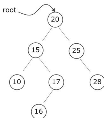
图 3-66 BST
