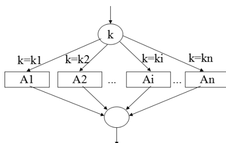
图 2.21 多路分支的逻辑
