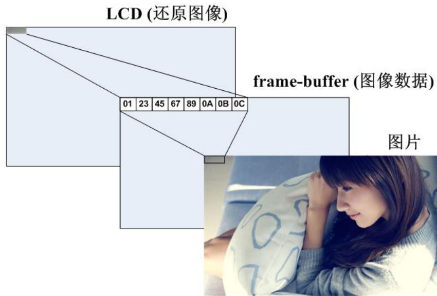
图 6-15 填充图片数据到映射内存
