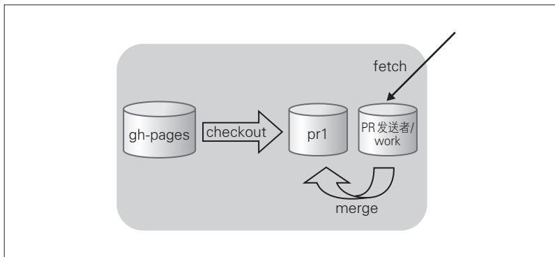
图 7.9 checkout
