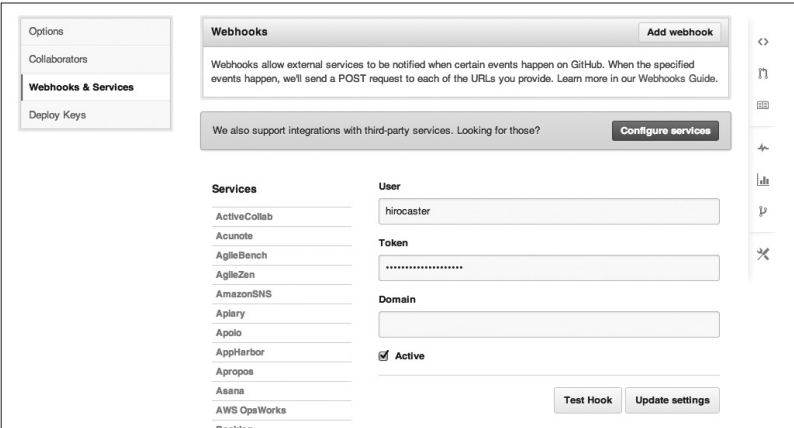
图 8.3 Hook 的测试
