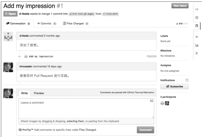
图 6.6 Pull Request
