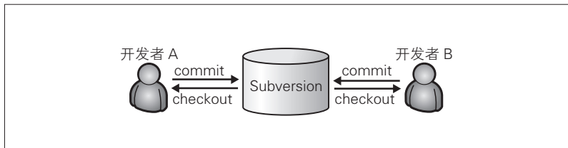
图 2.1 集中型
