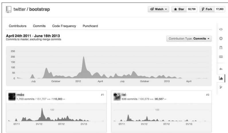
图 5.29 Contributors
