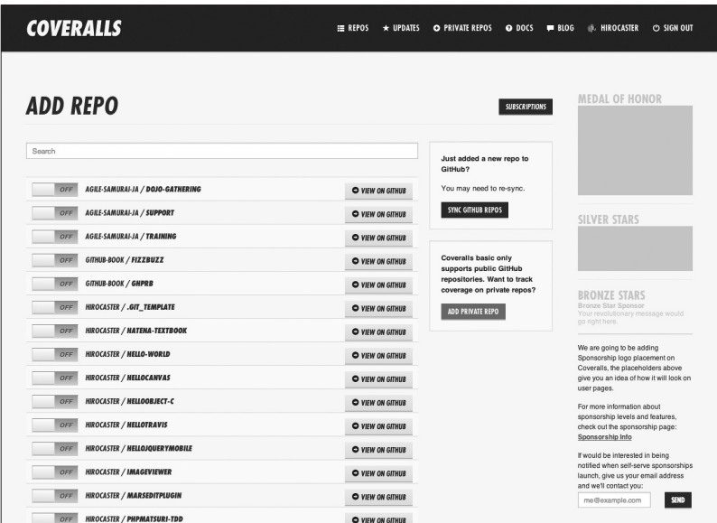
图 8.8 仓库列表
