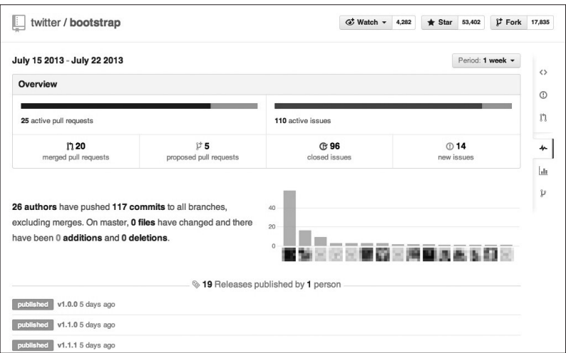
图 5.26 Pulse 的页面
