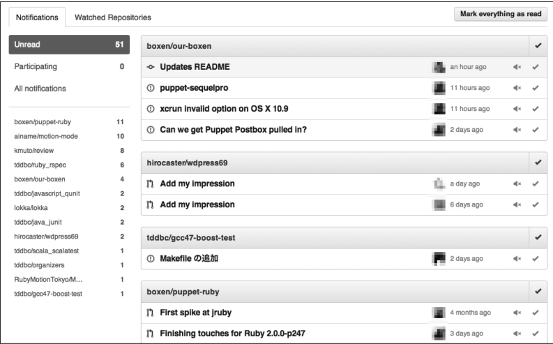
图 5.37 Notifications 的页面
