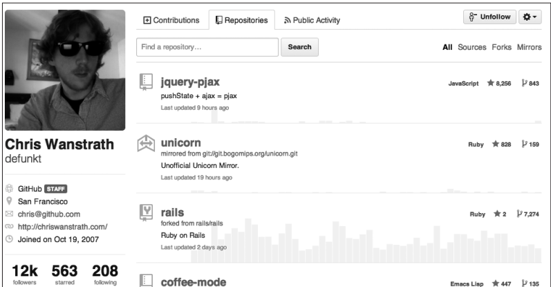
图 5.5 Repositories 标签页
