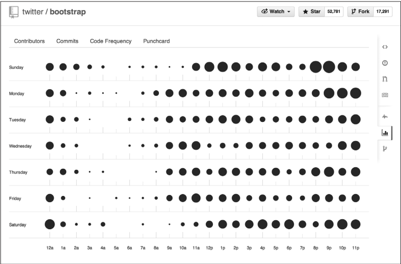
图 5.32 punchcard
