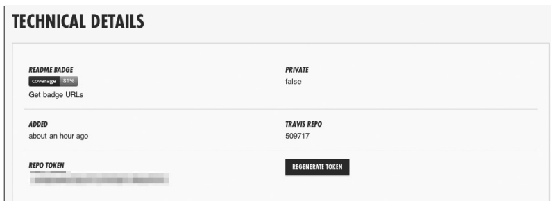
图 8.10 Coveralls 的标记
